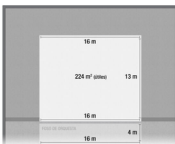
AUDITORIO Y PALACIO DE CONGRESOS EL BATEL SALA A. Plano planta del escenario
