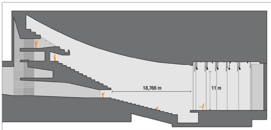
AUDITORIO Y PALACIO DE CONGRESOS EL BATEL SALA A. Plano longitudinal
